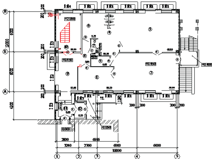
План 1-го этажа на ош. +0.450
