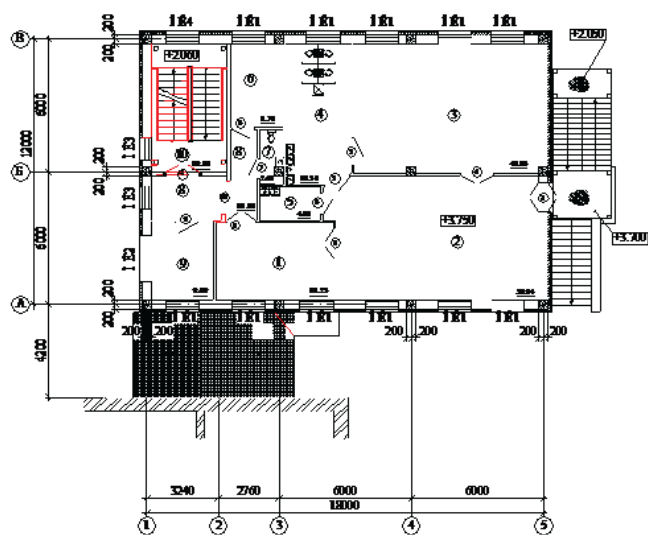
План 2-го этажа на ош. +3.750
