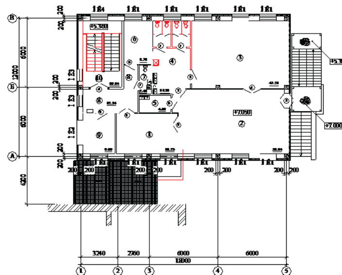
План 3-го этажа на ош. +7.050
